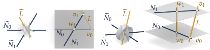
Fig. 24. Proof of Lemma A.1.
