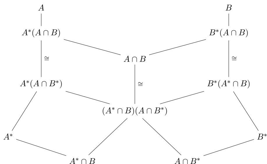
Abbildung 8.2: „Schmetterlingslemma“
